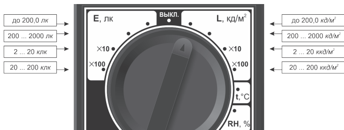
Рис.2 – Пределы измерения световых параметров
