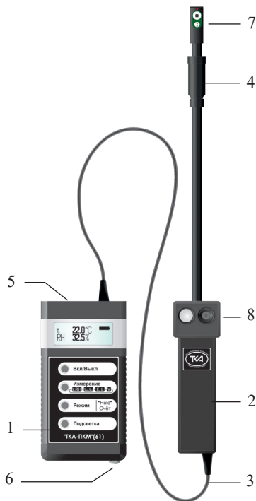
Рис.1 Внешний вид прибора “ТКА-ПКМ”(61)
