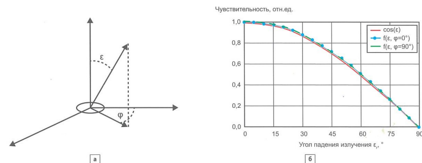
Рис. 3. а) система координат для определения пространственной чувствительности люксметра (по ГОСТ Р 8.850-2013); б) результат определения угловой чувствительности фотоприемного устройства конструкции НТП «ТКА» при государственных испытаниях средства измерений
