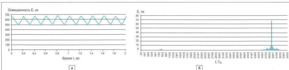
Рис. 4. а) осциллограмма типовой пульсации освещенности прибора; б) анализ гармоник пульсирующего светового потока. В диапазоне 0–300 Гц пульсация светового потока практически отсутствует
